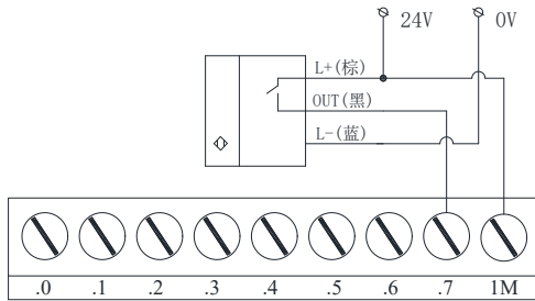
PNP型接近/霍尔开关接线示意图
